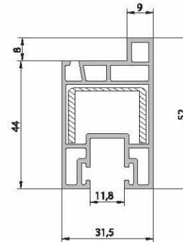
W-150 NAVE DOBLE CORREDERA CODIGO : 21313 - 05000
