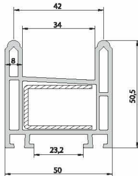
W-150 MARCO DOBLE CORREDERA CÓDIGO : 21313 - 01000
