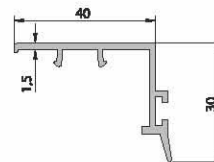
W - 150 TAPA ENGANCHE CÓDIGO : 20105 - 01100
