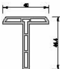
T PROFILE 21601 - 06000 : WHITE
