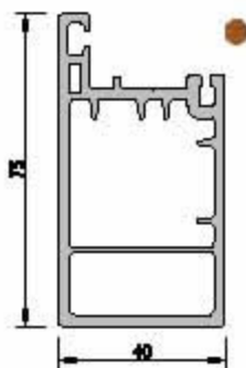
SASH PROFILE R.21601-01003 : ROBLE
