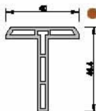
T PROFILE R.21601-06003 : ROBLE
